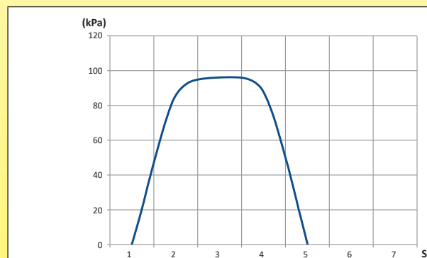
Grafico dell'aumento di pressione all'interno di un pulsante pneumatico di 32 mm di diametro (come il modello 66ZM5 descritto in questo catalogo)
